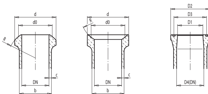
KF-Kugel Schott
